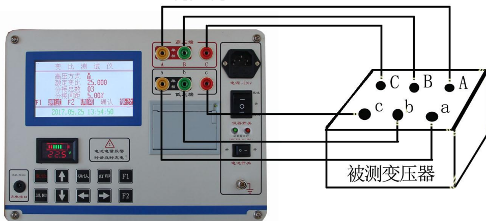
图 10 三相变压器变比测试接线图
