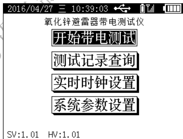
图7 主菜单
