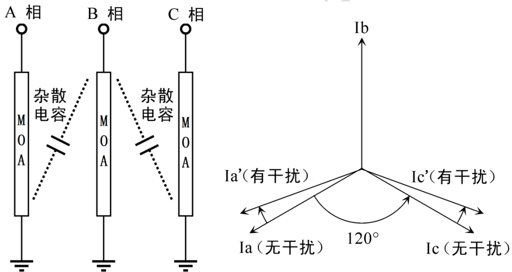
图 2 相间干扰
