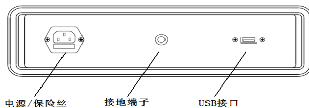
图 1b 变压器绕组变形测试仪后面板图(后面板)
